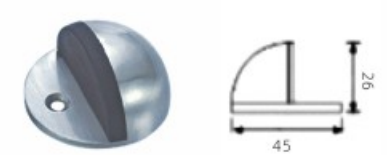
HSP114 SN GP AB AC BLK
