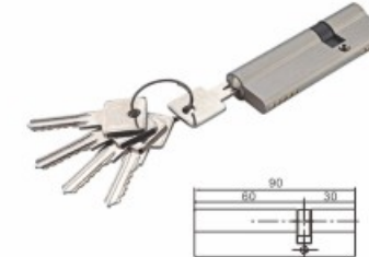
B90MM-UN(30MM+60MM) COLOR : SN
