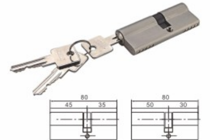
B80MM-UN(35MM+45MM) B80MM-UN(30MM+50MM) COLOR : SN
